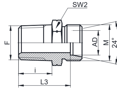
接头体
