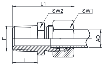
卡套式接头
