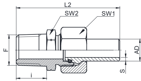
焊接式接头
